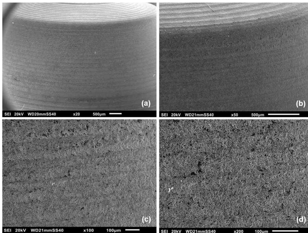
Figura 14 - Punção 2 novo; (a) imagem de elétron secundário com aumento de 20 vezes; (b) 50 vezes; (c) 100 vezes; (d) 200 vezes
