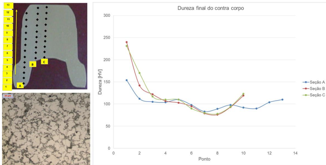
Figura 20 - Dureza e microestrutura da peça após a 2ª operação
